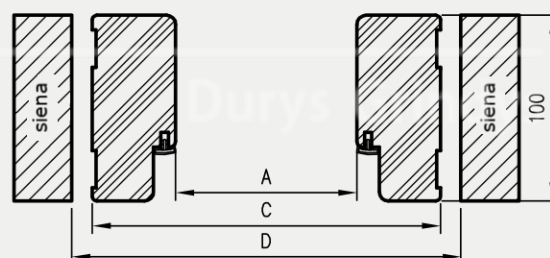
Detalūs pločio matmenys
