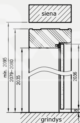
Detalūs aukščio matmenys durims su stikline varčia
