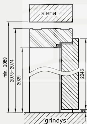
Detalūs aukščio matmenys durims su užlaida
