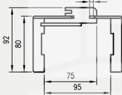
Dvivėrėms durims
