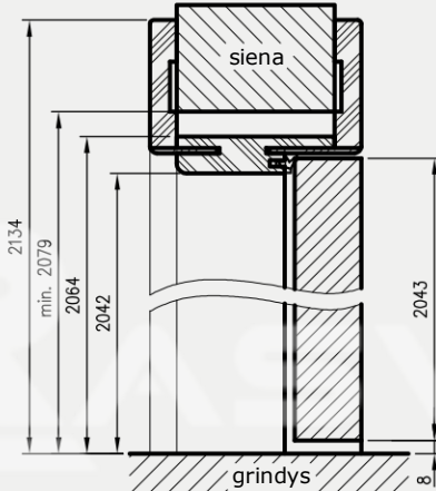
Detalus aukščio matmenys lygiabriaunėms durims
