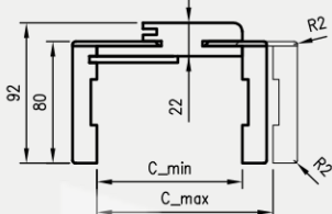
Detalus pjūvis 075mm gaubimo staktai
