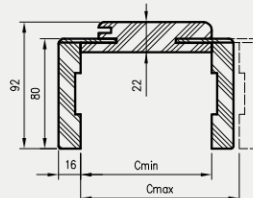
Detalūs pločio matmenys
