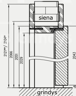
Detalus aukščio matmenys stiklinėms durims
