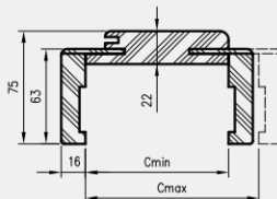
Detalus pjūvis T63 staktai
