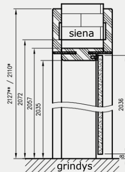
Detalus aukščio matmenys stiklinėms durims
