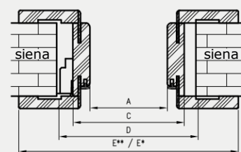
Detalūs pločio matmenys
